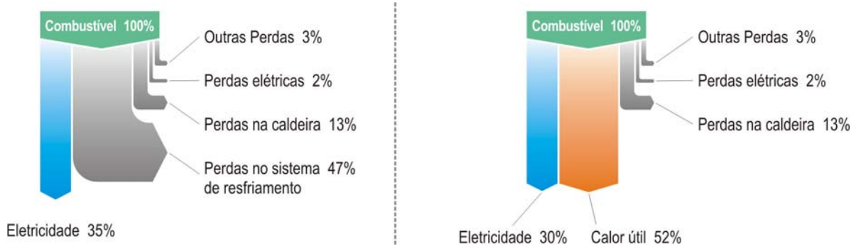
Figura 2-11 a) Balanço térmico típico de planta de geração pura, em ciclo a vapor; b) Balanço térmico de uma planta semelhante, com sistema de cogeração agregado (adaptado de NOGUEIRA et al., 2004) [70] .
