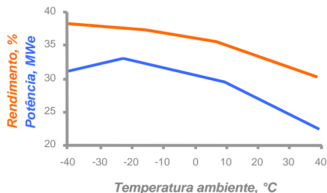
Gráfico 2-2 Influência da temperatura do ar ambiente em turbinas a gás ( Rolls-Royce Energy Systems, 1998 ).
