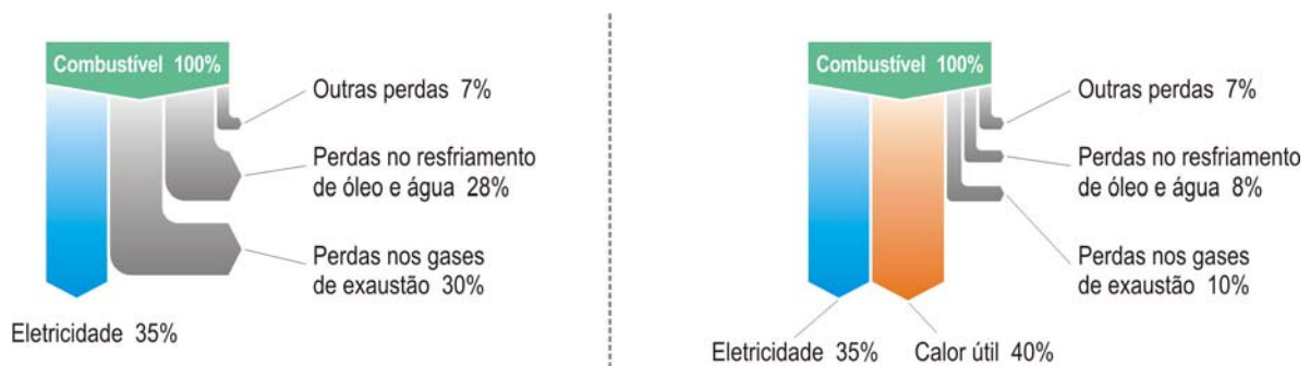
Figura 2-18 a) Balanço térmico típico de planta de geração pura utilizando motor alternativo; b) Balanço térmico de uma planta semelhante, com sistema de cogeração agregado (adaptado de NOGUEIRA et al., 2004) [10] .
