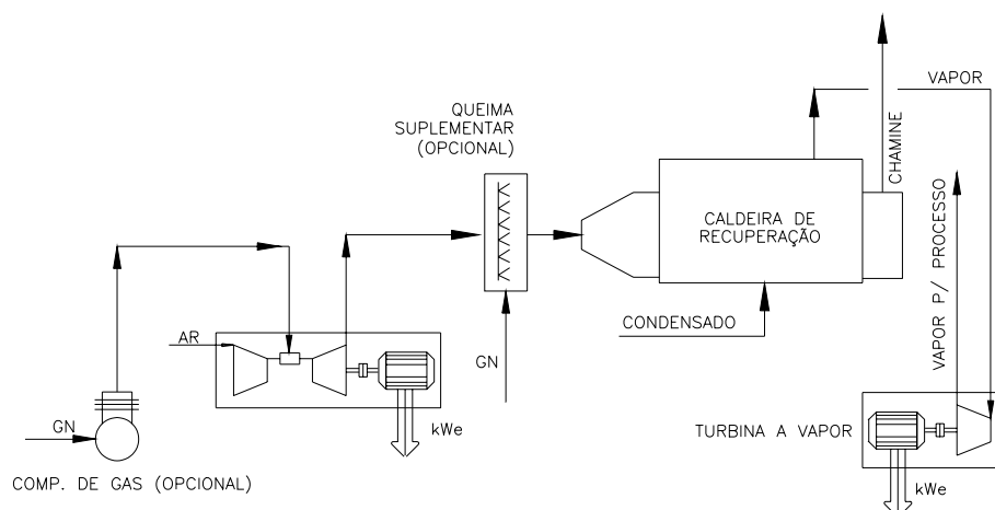
FIGURA 3 – Sistema de co-geração com turbinas a vapor e turbinas a gás
