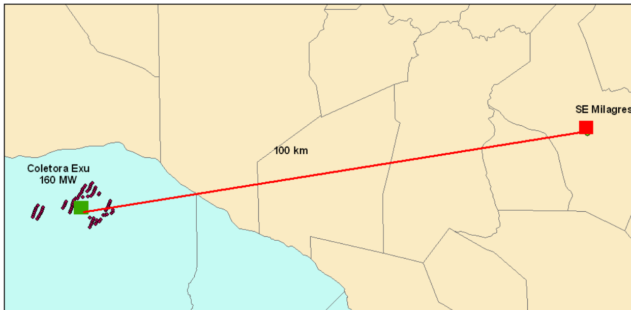
Figura 4-5 Esquema de conexão da coletora Exu - Pernambuco
