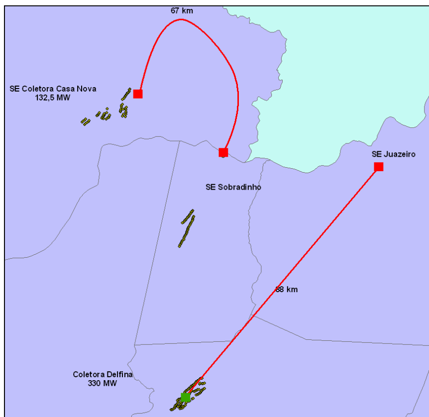
Figura 4-6 Esquema de conexão da Coletora Casa Nova – Bahia
