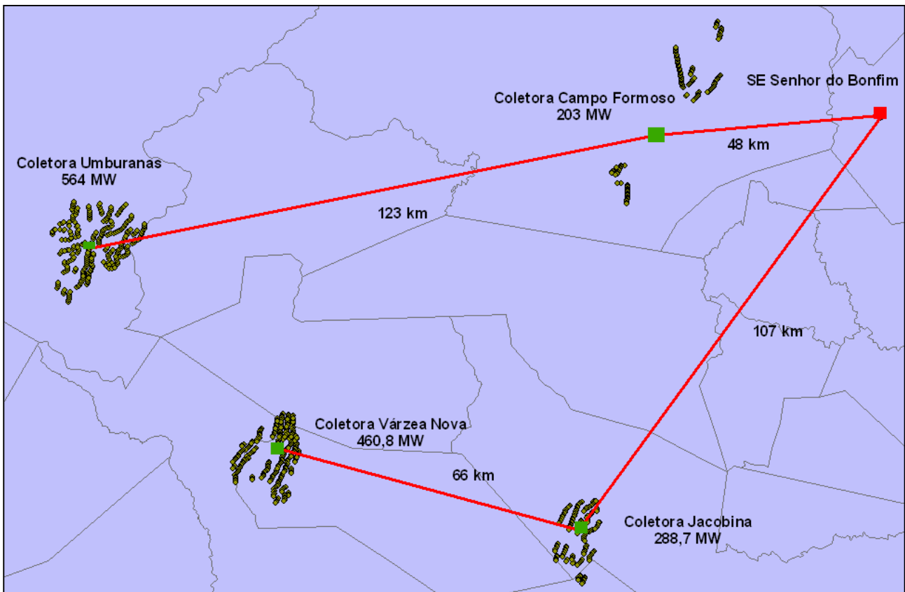
Figura 4-7 Esquema de conexão das Coletoras Campo Formoso, Umburanas, Jacobina e Várzea Nova
