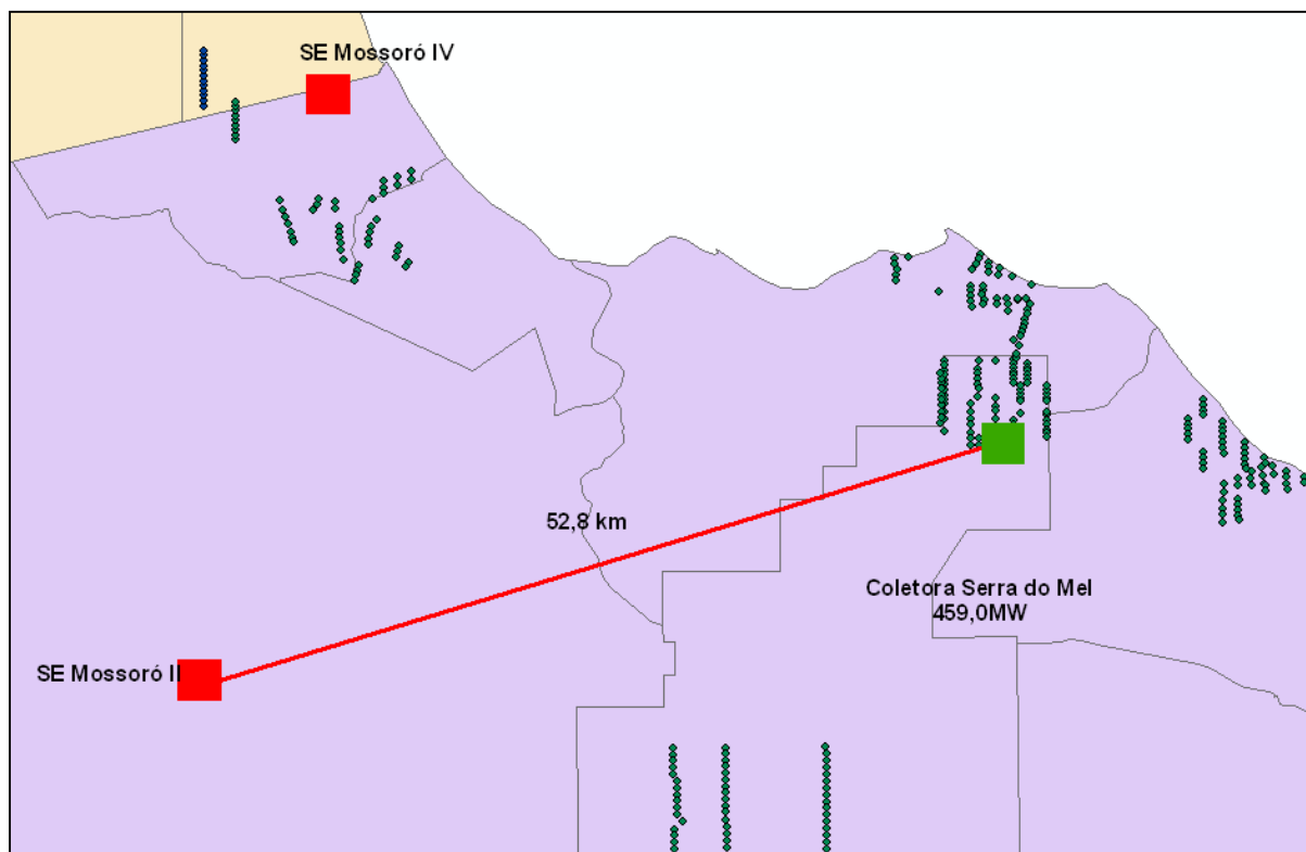
Figura 4-1 Esquema de conexão da coletora Serra do Mel – Rio Grande do Norte
